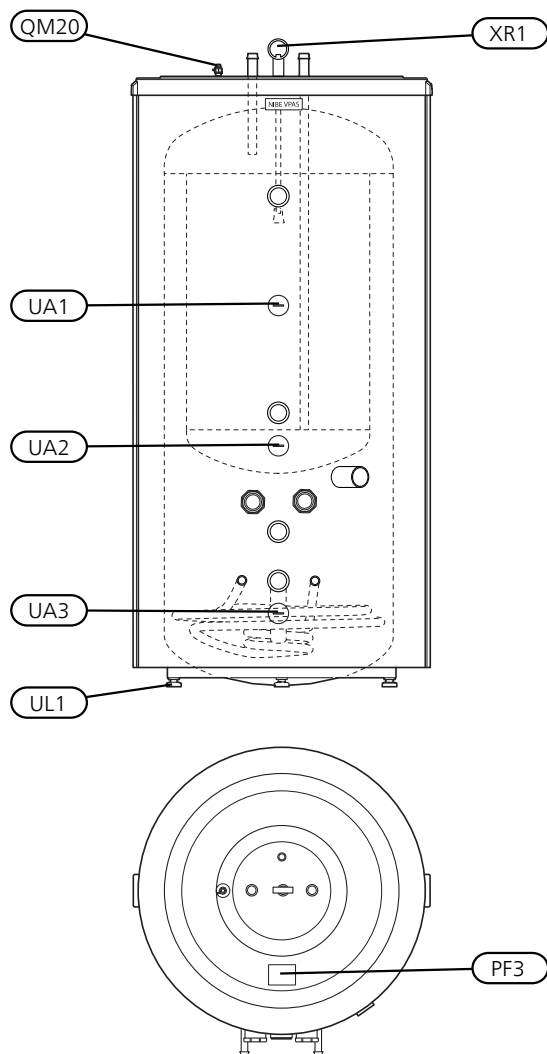
VPAS 300/450 -Cu
