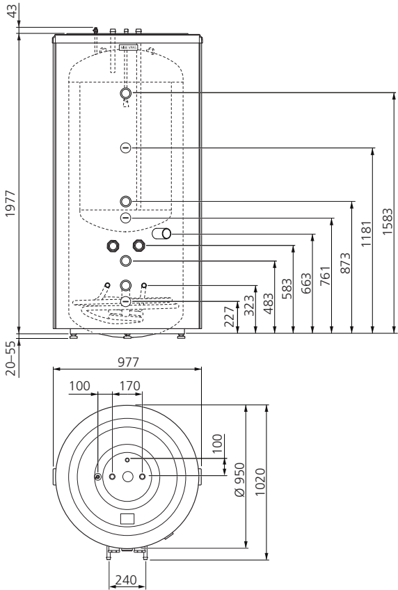
VPAS 300/450 -E
