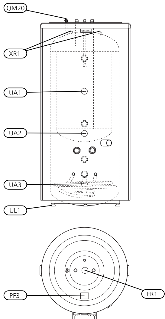
VPAS 300/450 -E
