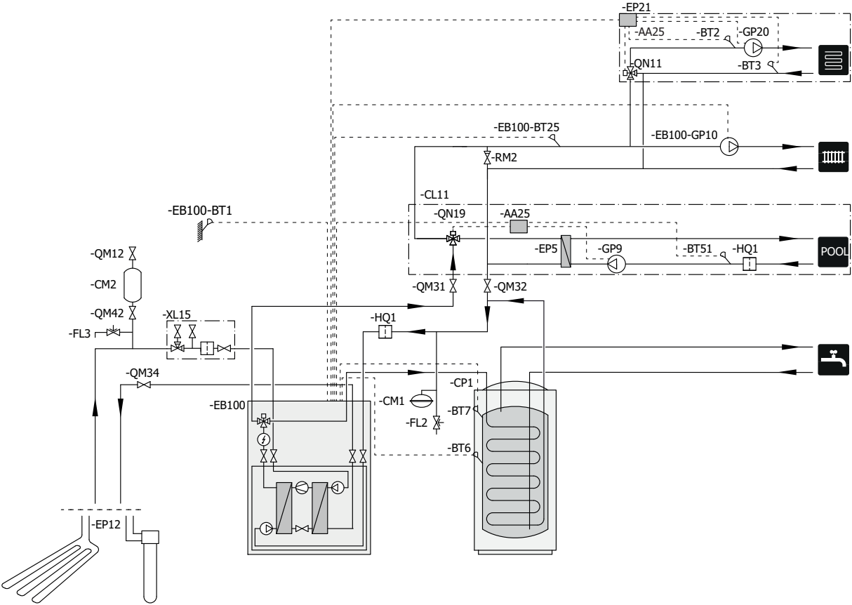
Principschema F1145/F1155 med POOL 40 och extra klimatsystem
